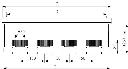
Возможные варианты исполнения светильников ДСО11-920, 921, 922, 923, 924
