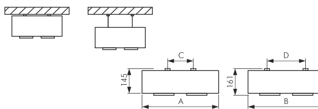
Возможные варианты исполнения светильника ДПО11-920,924
